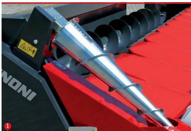
1 BOCZNE ŚLIMAKI STOŻKOWE Боковые конические вальцы Konusni spiralni bočni valjci Странични винтови делители
