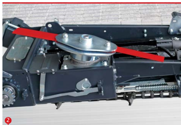
2 ROZDRABNIACZ ŁODYG Измельчитель Sečka Раздробителите на стъбла
